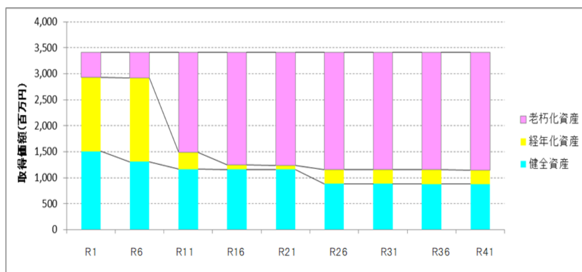
図-4.3 (1) 更新を行わなかった場合の健全度（施設及び設備）
