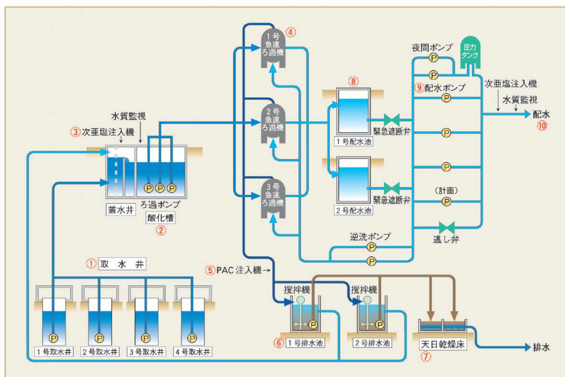
山武浄水場（平成 12 年竣工）
