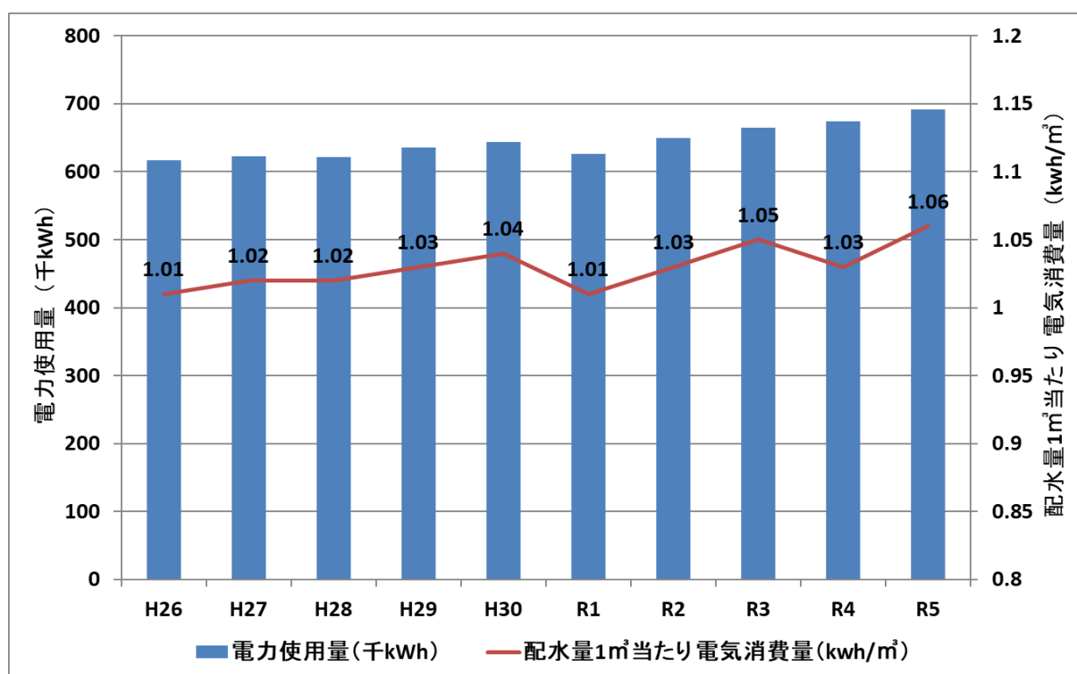
図-3.10 電力使用量等の推移
