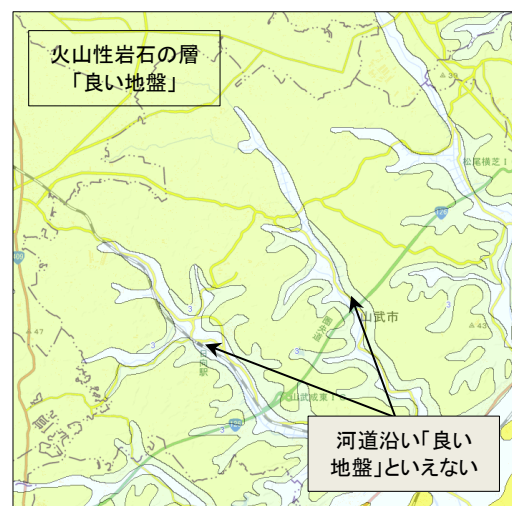
図-3.2 山武地域の地質
