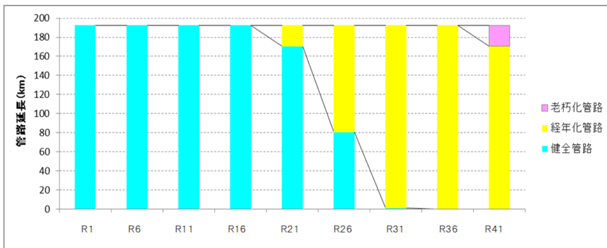
図-4.3（2） 更新を行わなかった場合の健全度（管路）
