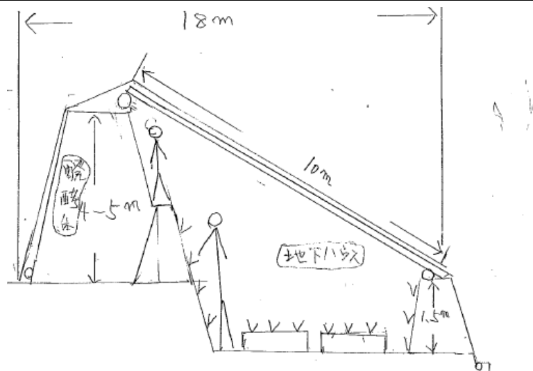
※醗酵暖房機付き地下ハウスの図面
